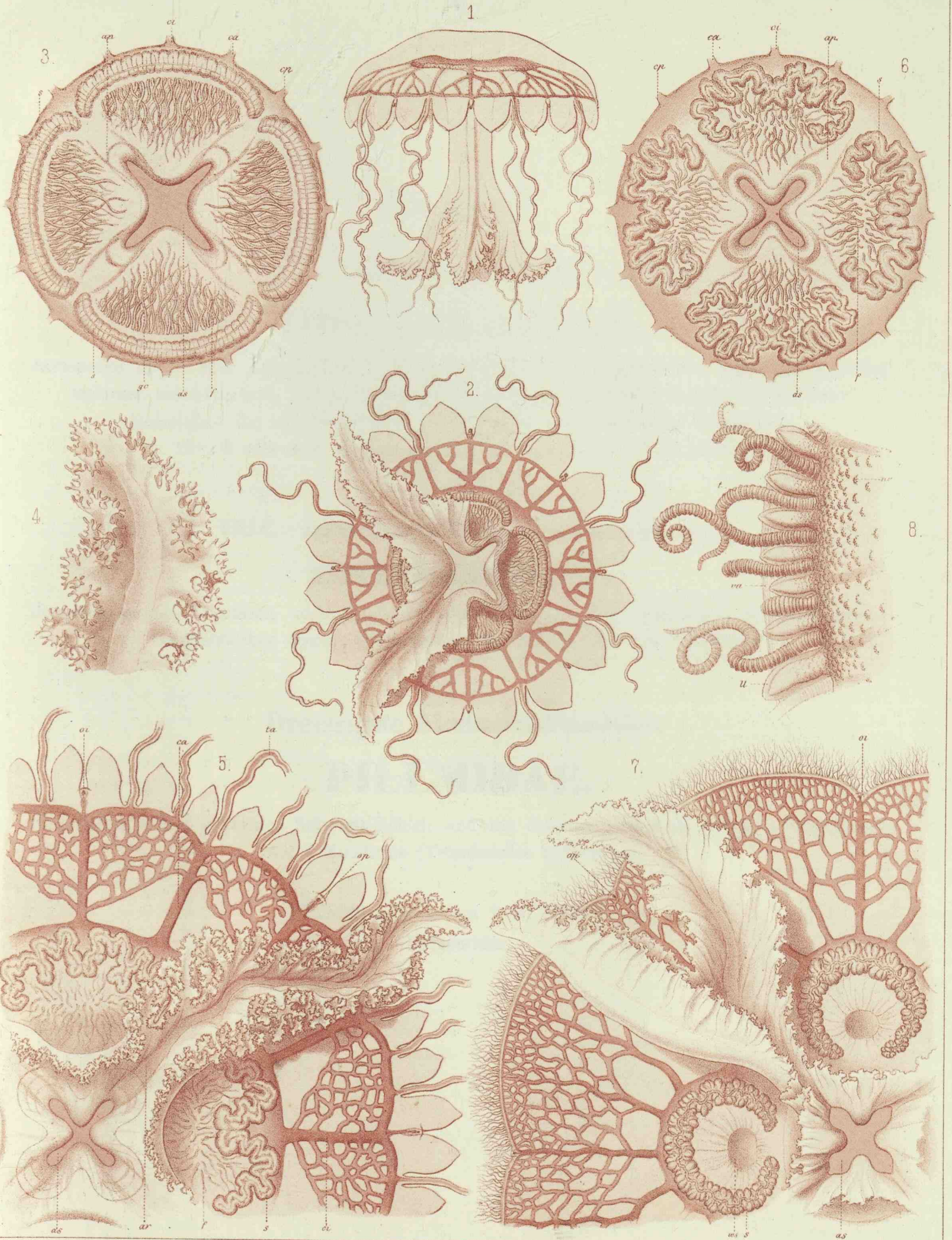
1-4. ULMARIS, 5, 6. UNDOSA, 7, 8. AUROSA.
