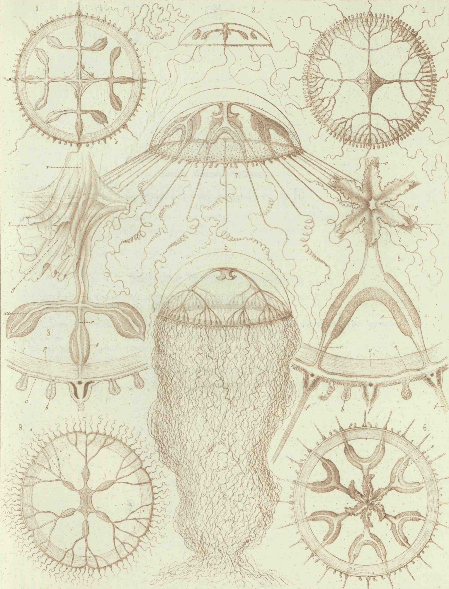
1-3. STAURODISCUS, 4, 5. BERENICE, 6-8. TOXORCHIS, 9. DIPLEUROSOMA.
