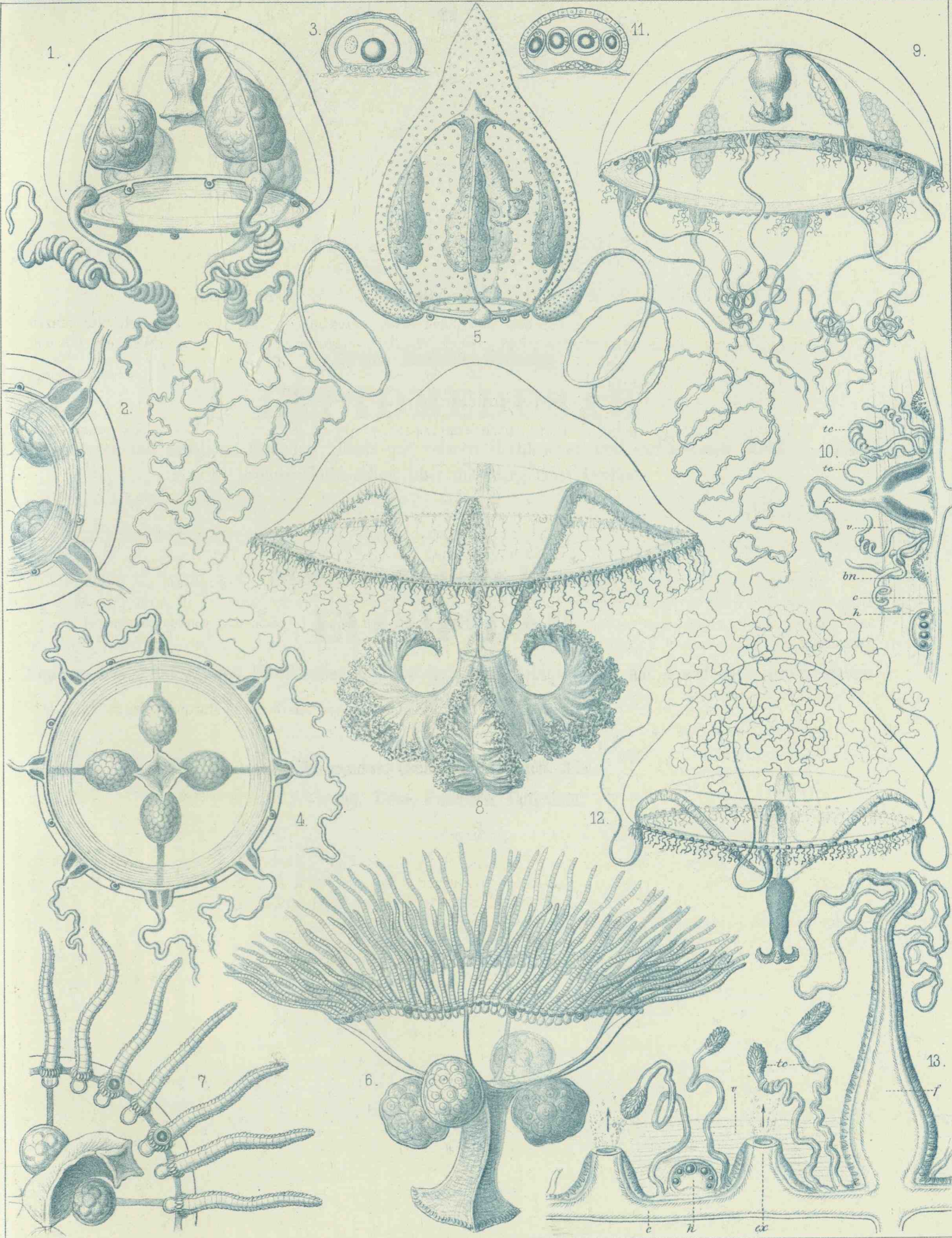
1-3. EUCOPIUM, 4. EUCOPE, 5. SAPHENELLA, 6. 7. OBELIA, 8. EUTIMALPHES, 9-11. MITROCOMIUM, 12. 13. JRENIIUM.*
