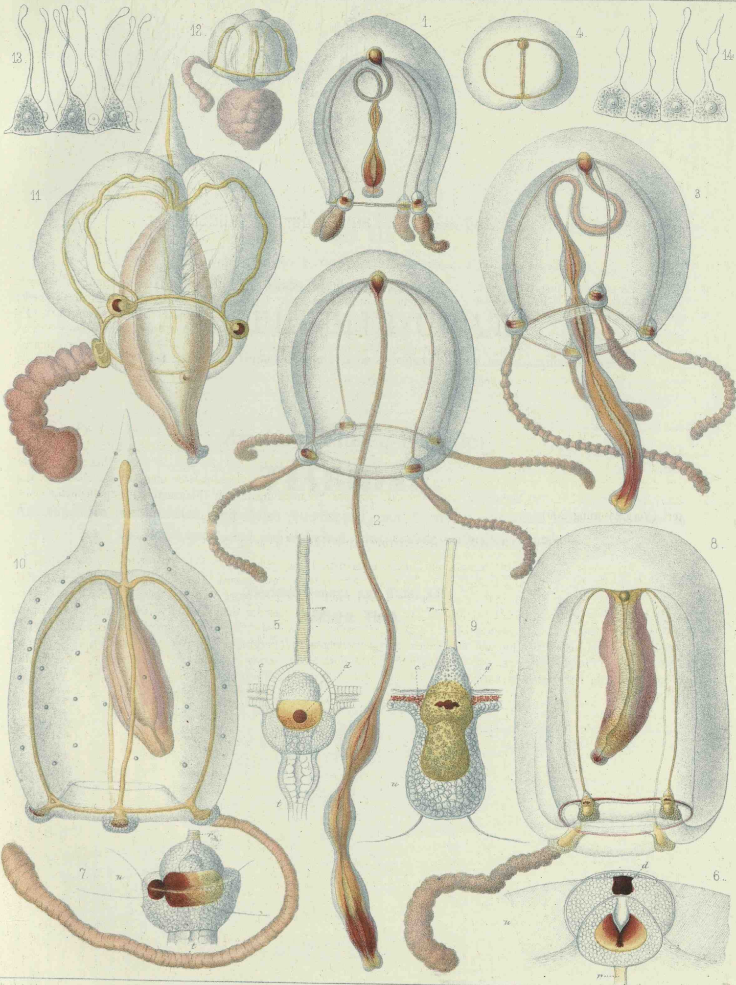
1-7. DIPURENA, 8-9. EUPHYSA, 10-14. STEENSTRUPIA.
