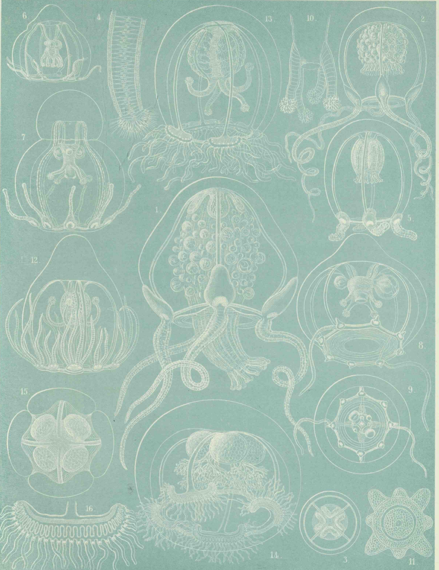
1-5 NIGRITINA, 6, 7 BLASTOGASTER, 8-11. CUBOGASTER, 12. LIZUSA, 13. MARGELLUM, 14-16. MARGELIS.
