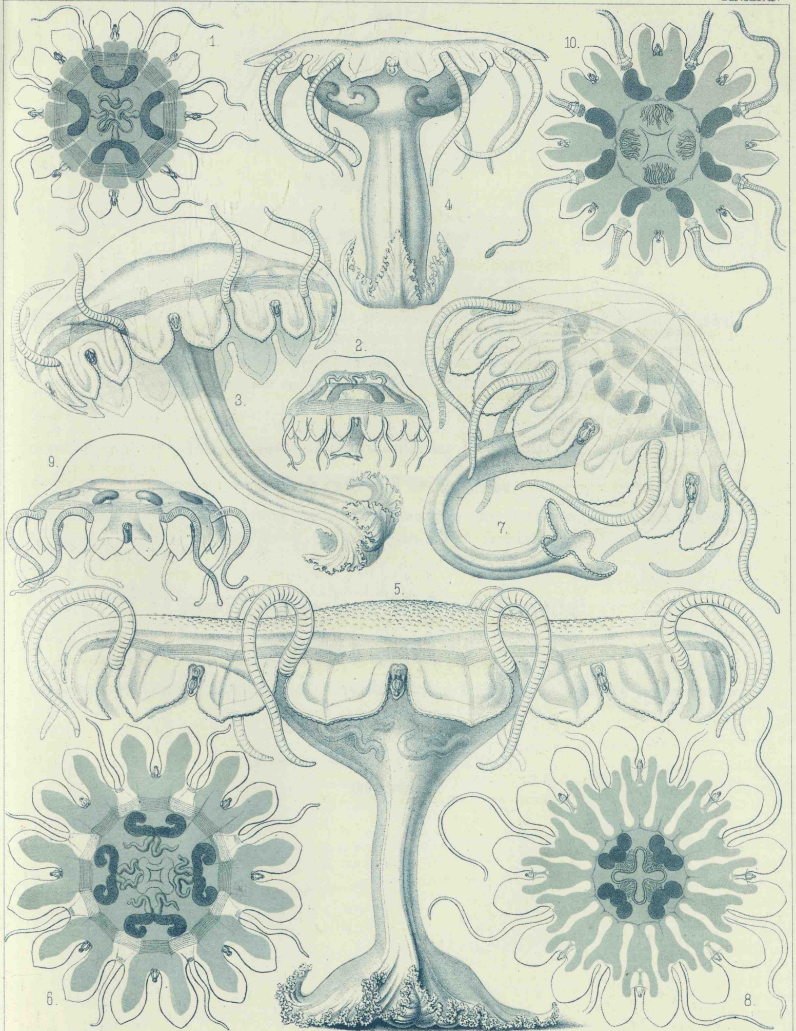
1. 2. EPHYRA, 3-6. PALEPHYRA, 7. 8. ZONEPHYRA, 9. 10. NAUSICAA.
