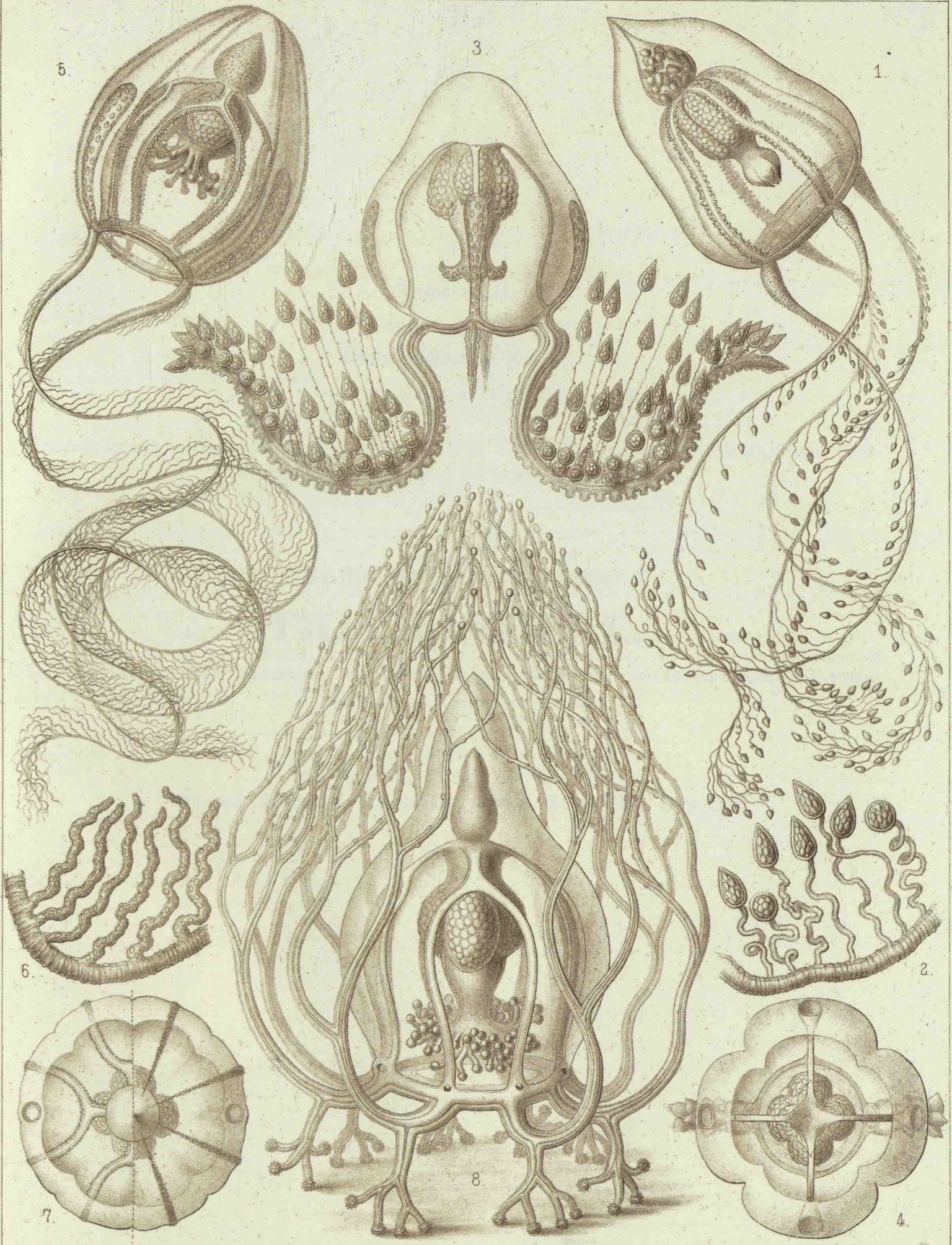
1. 2. PTERONEMA, 3. 4. GEMMARIA, 5-7. CTENARIA, 8. DENDRONEMA.
