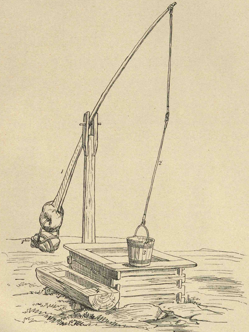
1. Cumpănă.—1 bis. Greutate (un buturug sau un bolovan).—2. Prăjină.— 3. Găleată sau cîtură.—4. Jghiab sau teucă.
