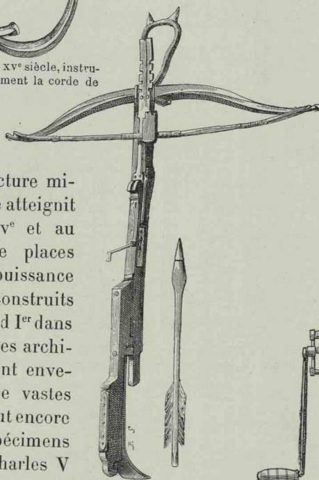
Grande arbalète à tour de siège du XV e siècle.
