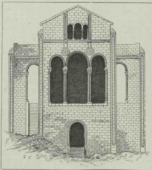
Église de Santa Maria de Naranca (province d'Oviédo), considérée comme le palais de don Ramire (842-850) et comme ayant été édifée au milieu du ix e siècle (Monumentos arquitectonicos).
