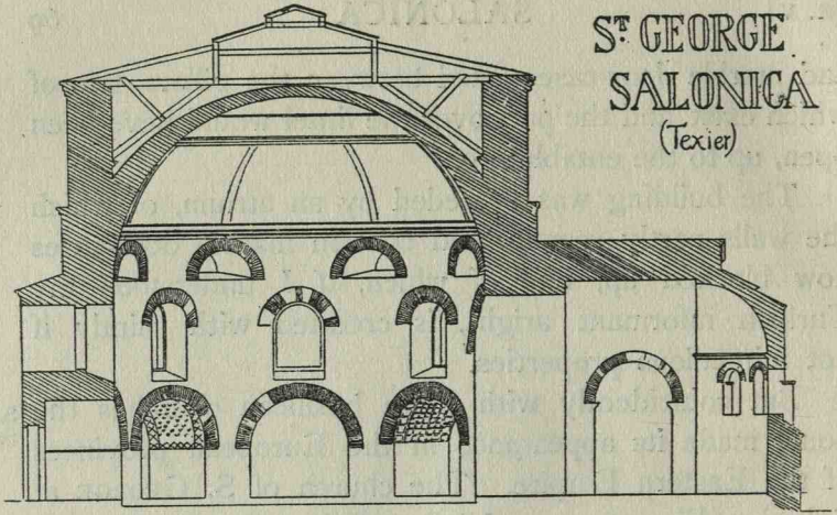
LONGITUDINAL SECTION
