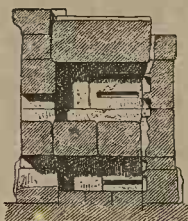
Fig. 194. — Le Burdj-el-Bezzâk. Coupe (d'après Renan).
