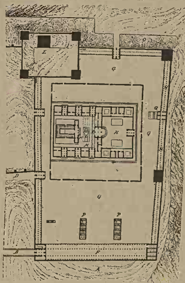
Fig. 168. — Plan du temple d'Hérode (d'après M. de Vogüé) 1 .
