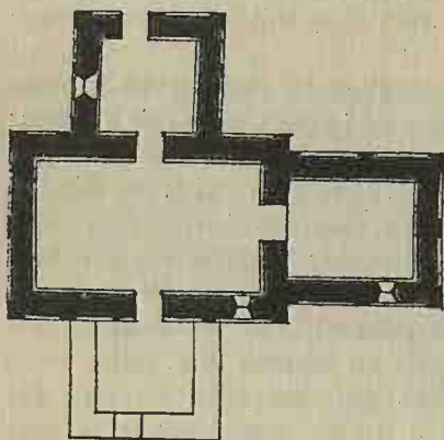
Abb. 181. Bradford-on-Avon.
