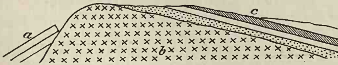
a geschleppte Scholle. b Rumpfscholle. c transgredierende Tafelscholle.
