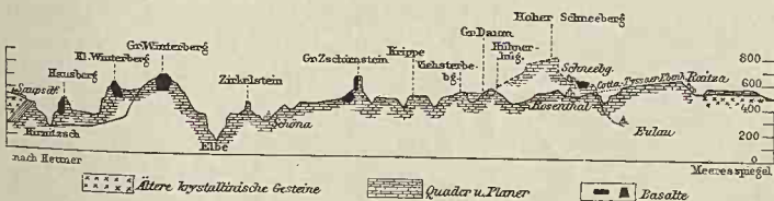
Geologisches Profil durch die sächsisch-böhmische Schweiz.
