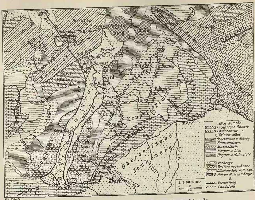
Tektonische Skizze des südwestlichen Deutschlands.
