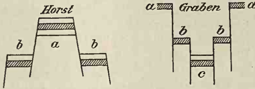
a Hochschollen. b Staffeln. c Tiefschollen.
