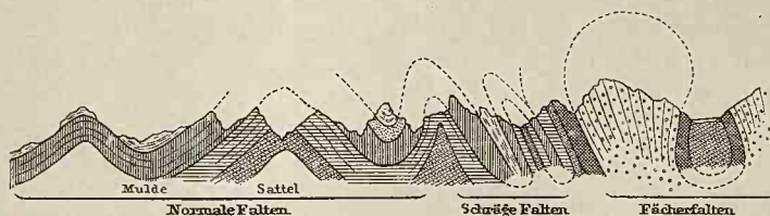
Schematische Skizze eines Faltengebirges.
