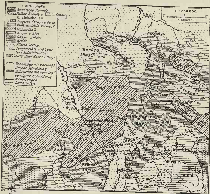
Tektonische Skizze der Rheinlande, Hessens und der Wesergebirge.
