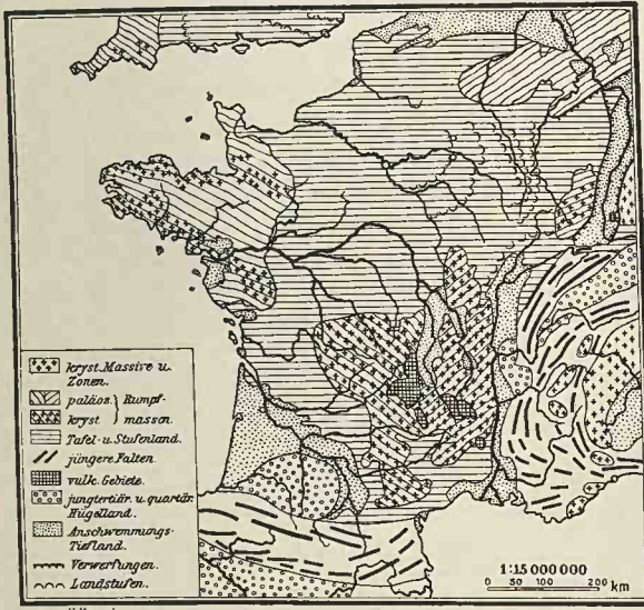
Tektonische Skizze.
