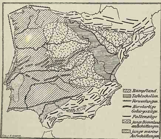
Tektonische Skizze.
