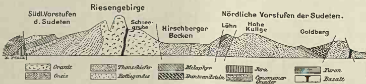
Geologisches Profil durch das Riesengebirge.
