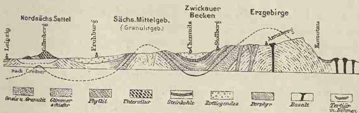
Profil durch die westsächsischen Gebirge.
