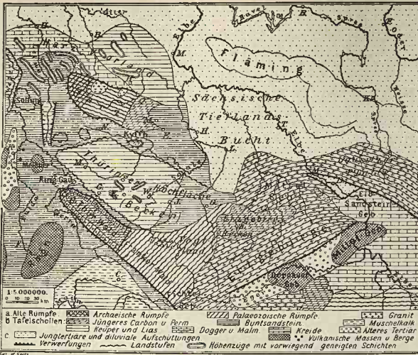
Tektonische Skizze von Thüringen und Sachsen.
