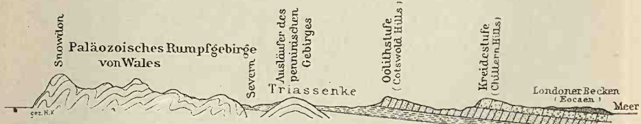
Geologisches Profil durch England.
