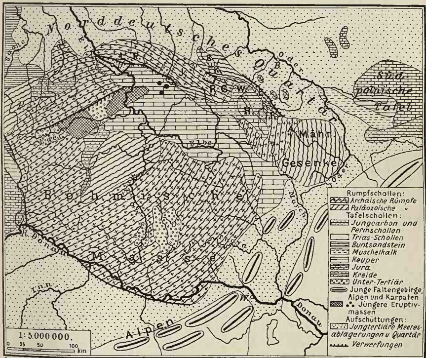
Tektonische Skizze von Böhmen und Mähren.
