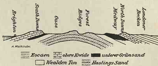
Geologisches Profil durch das Weald.
