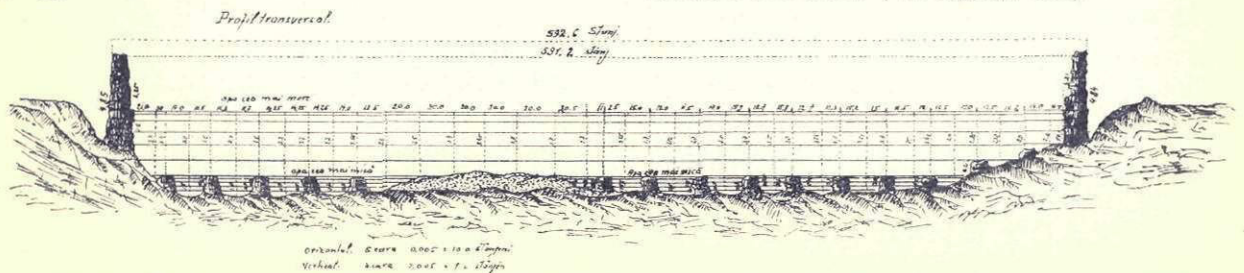
Fig. 9.—Planul transversal al rămășițelor podului lui Traian, studiate de ing. E. A. Popovici în Ianuarie 1858
