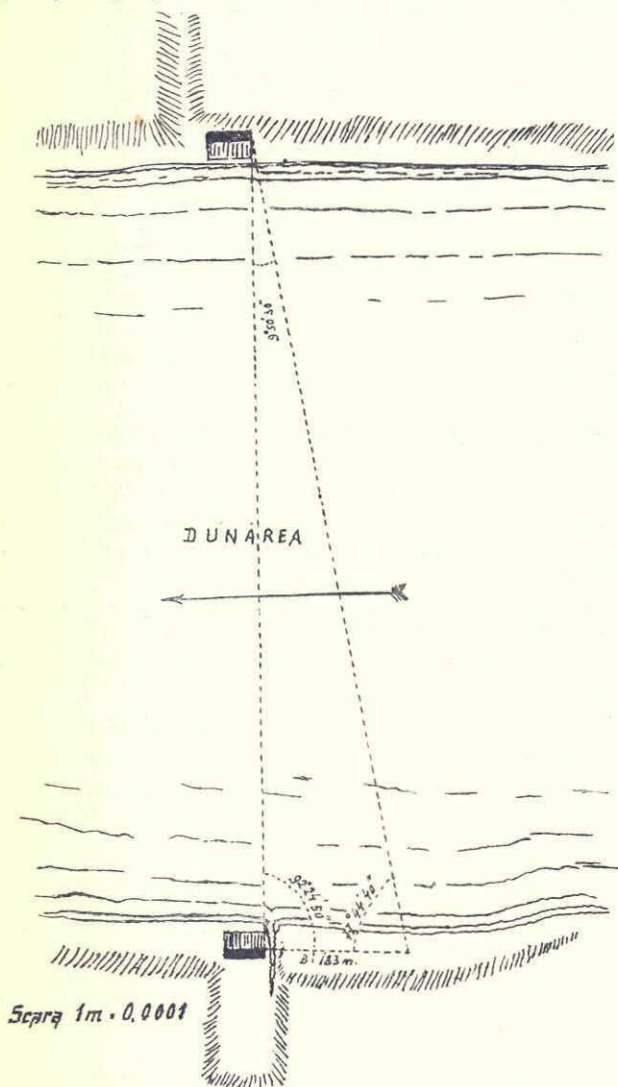
Fig. 10.—Măsurătoarea prin triangulație a lățimii Dunării la podul lui Traian, făcută la 17 Octombrie 1931
