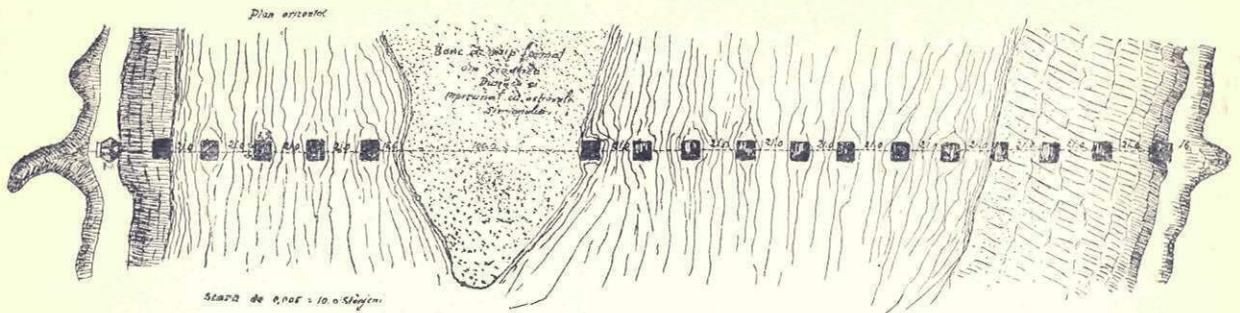
Fig. 8.—Planul orizontal al rămășițelor podului lui Traian, constatăte de ing. E. A. Popovici în Ianuarie 1858.
