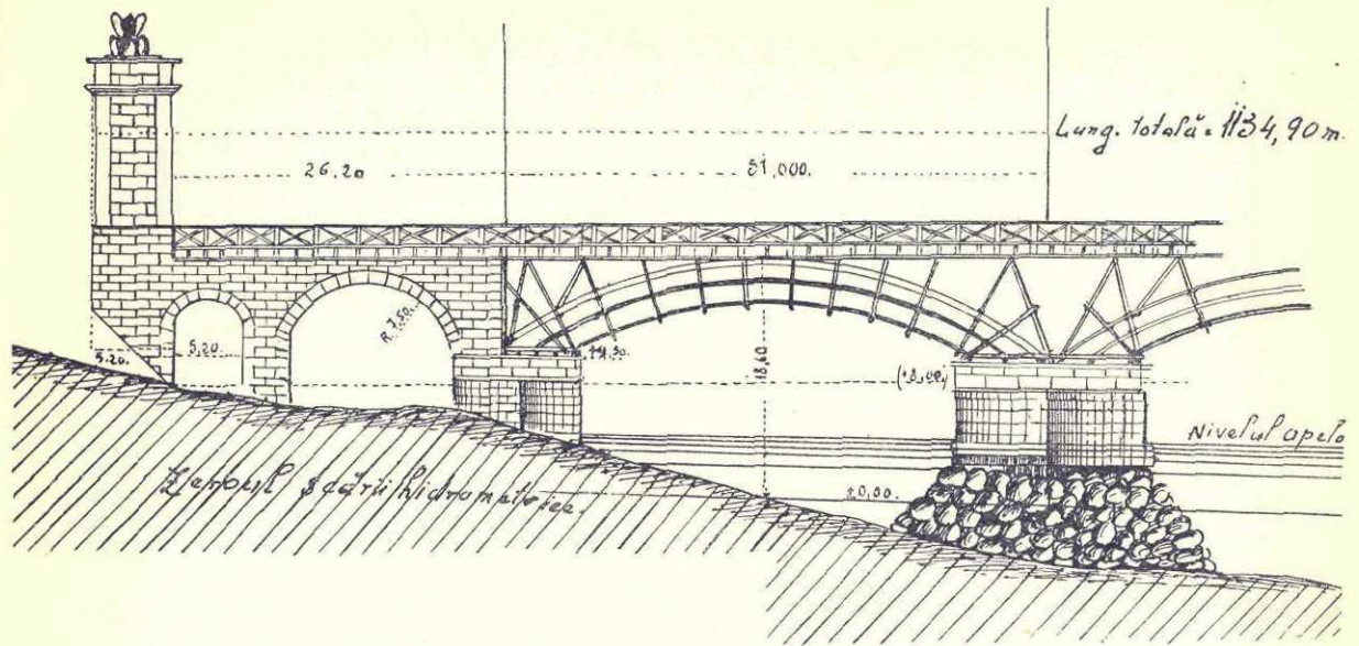
Fig. 14—Reconstituirea podului lui Traian de E. Duperrex : Portalul și prima boltă a podului la Drubeta
