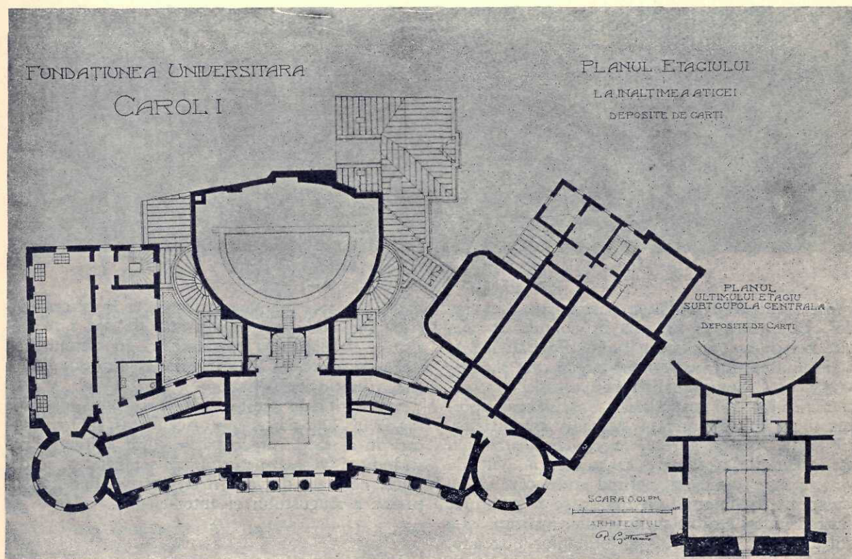
Planul depozitului de cărți al bibliotecii
