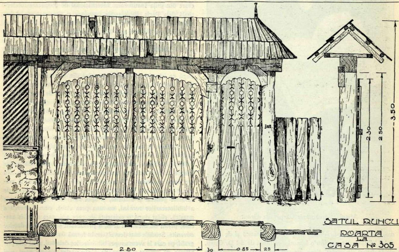
Poarta casei 305 din Runc, în schiță. (Din: H. H. Stahl, Tehnica , etc.)
