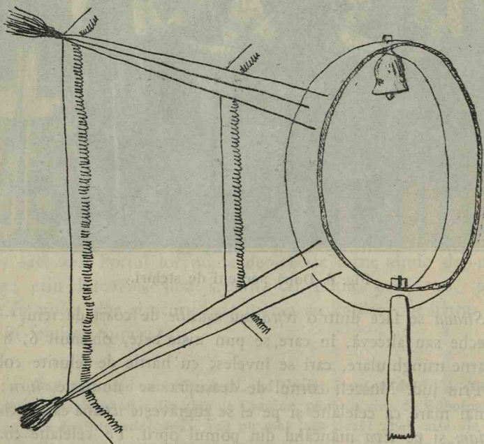
Fig. 7. Alcătuirea unei stele.
