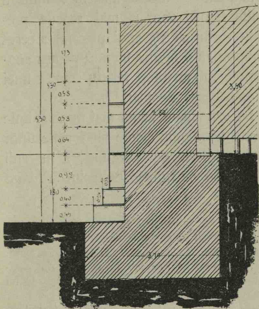
Fig. 3. Secțiune prin zidul cetății (archit. Fakler).
