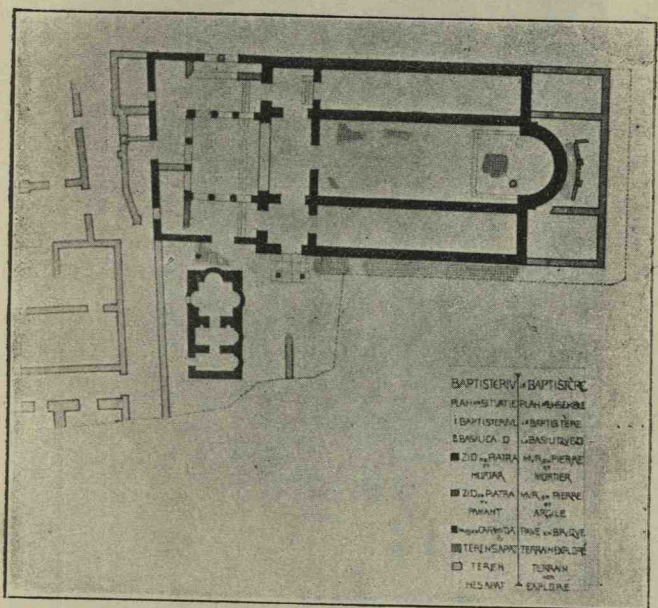
Fig. 20. Planul orizontal al basilicii de marmură, cu baptisteriul și clădirile târzii înconjurătoare (archit. Cegăneanu).
