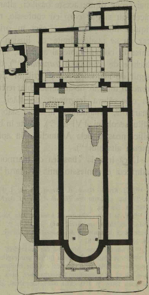
Fig. 15. Plan orizontal al basilicei de marmoră (Dr. ing. G. v. Cuibe).
