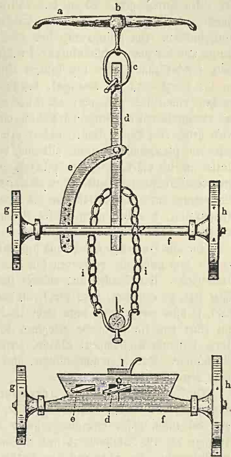
Fig. 104. Hölzerner Pflug älterer Art. Dat vortüg oder dat stell, Ansicht von oben und von hinten.
