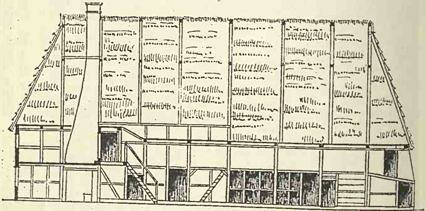
Fig. 58. Längsschnitt eines Hauses in Welpke von 1678. 1894 abgebrochen; bei a die nach der Däle zu offenen Ställe.
