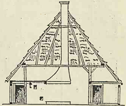
Fig. 61. Querschnitt.
