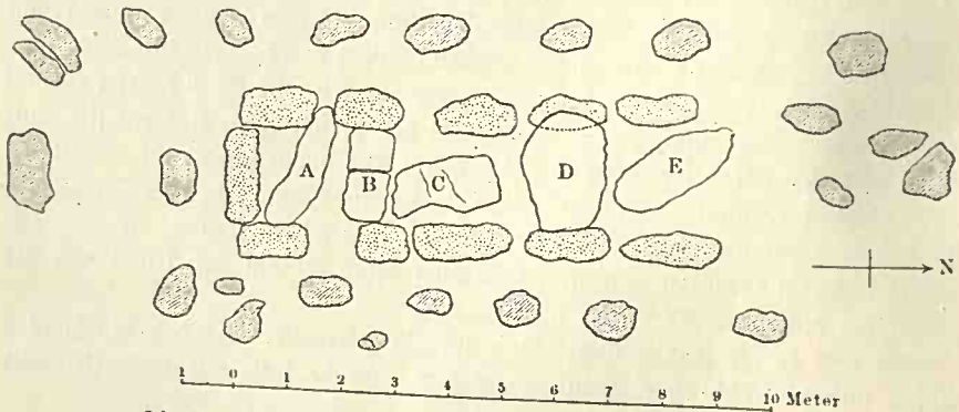
Fig. 3. Plan des großen Steinkammergrabes der Lösssteine.
