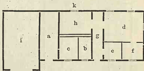
Fig. 89. Schulenrode Nr. 7 von 1769 (Etklof), typisch für viele Schulenroder Häuser.
