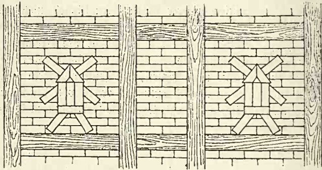
Fig. 70. Barnsteinsetzung, Wendeschott.
