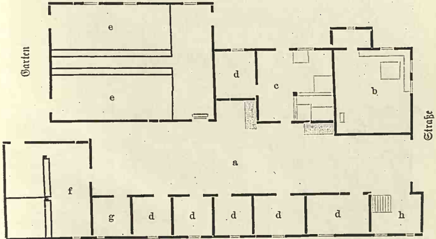
Fig. 69. Haus in Glentorf Nr. 27 (Warnecke). Grundriß.
